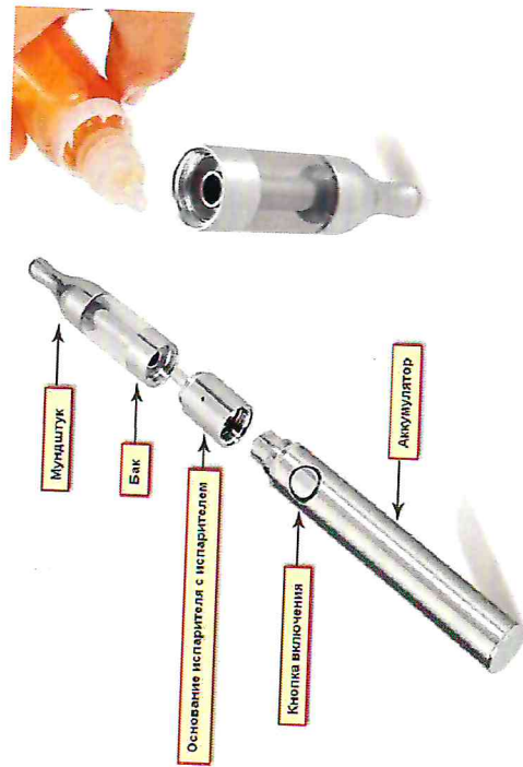
Рис. 3. Устройство электронной сигареты
